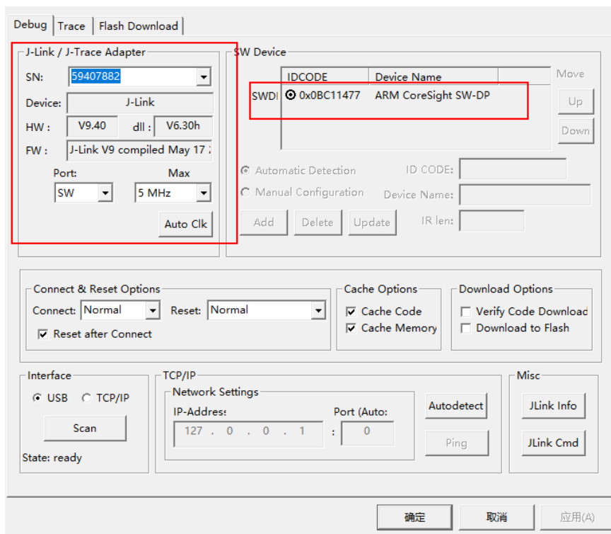
图 2-5: Debug 配置
