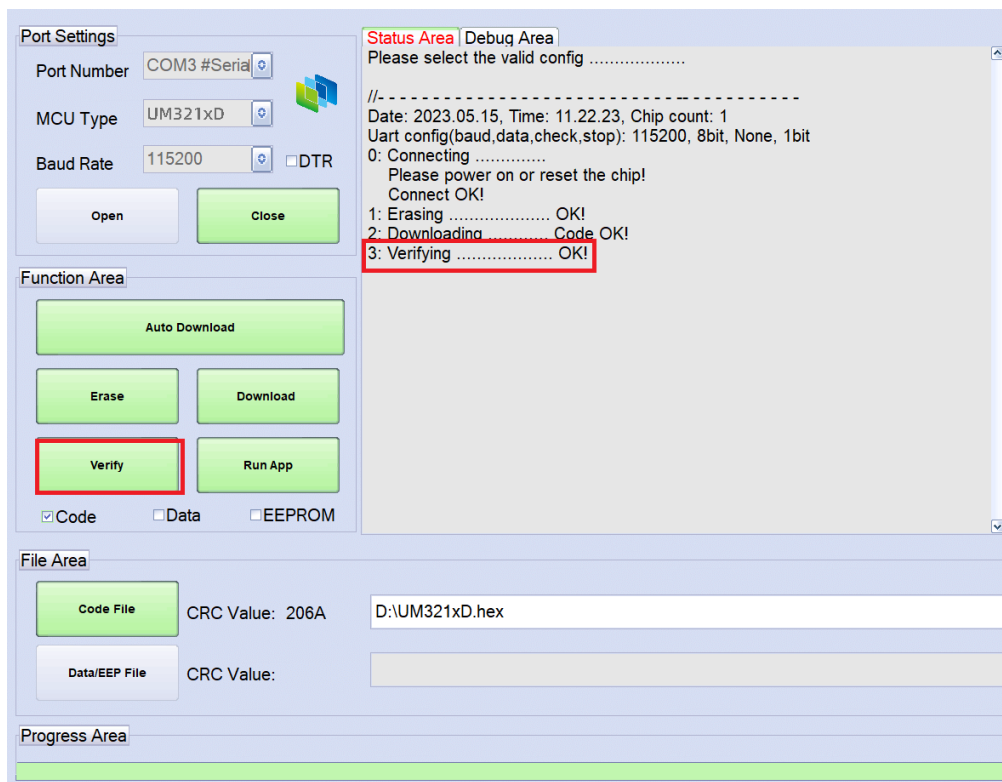
图 2-18: Verify 界面
