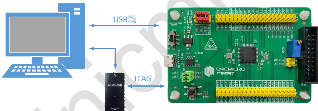
图 1-1：芯片开发硬件连接示意图
