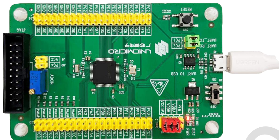
图 2-10：量产环境硬件示意图
