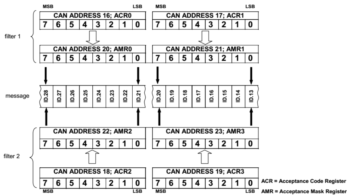
图 15-4：Dual filter for extended frame message
