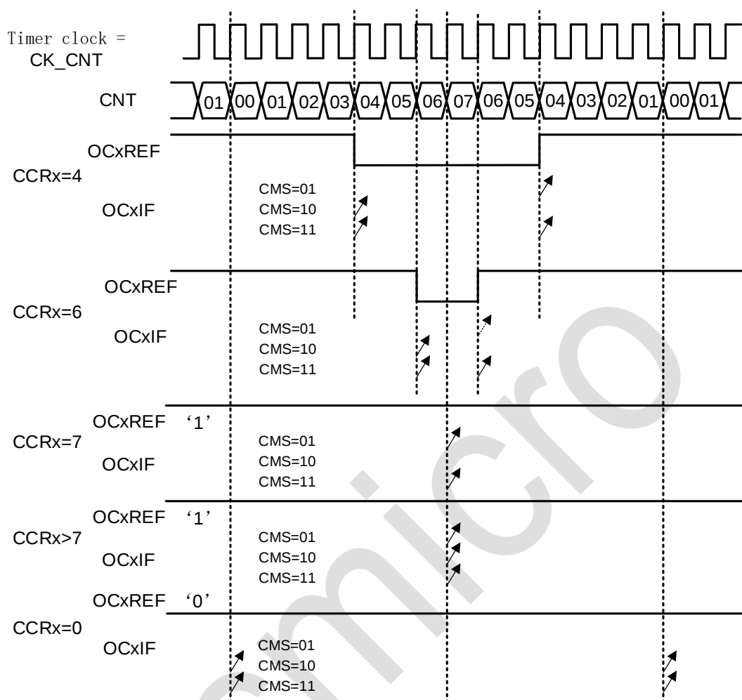
图 13-3: 中央对齐的 PWM 波形(APR=7)
