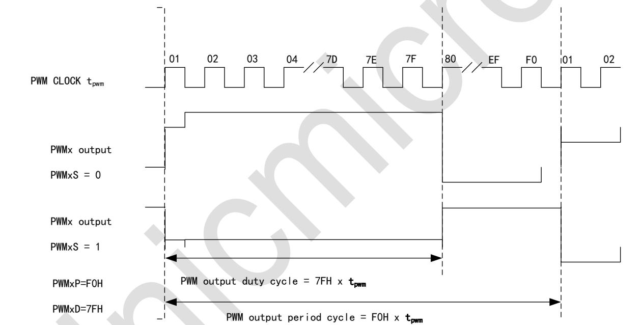
图 6-1：PWM 输出范例
