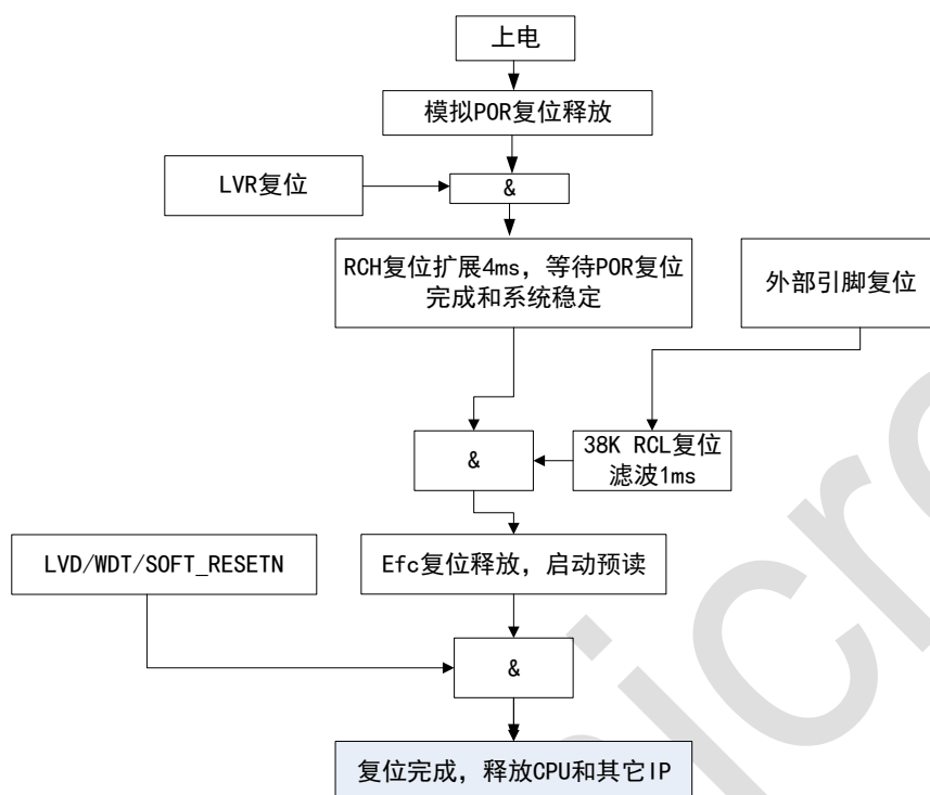
图 4-2: 复位流程图
