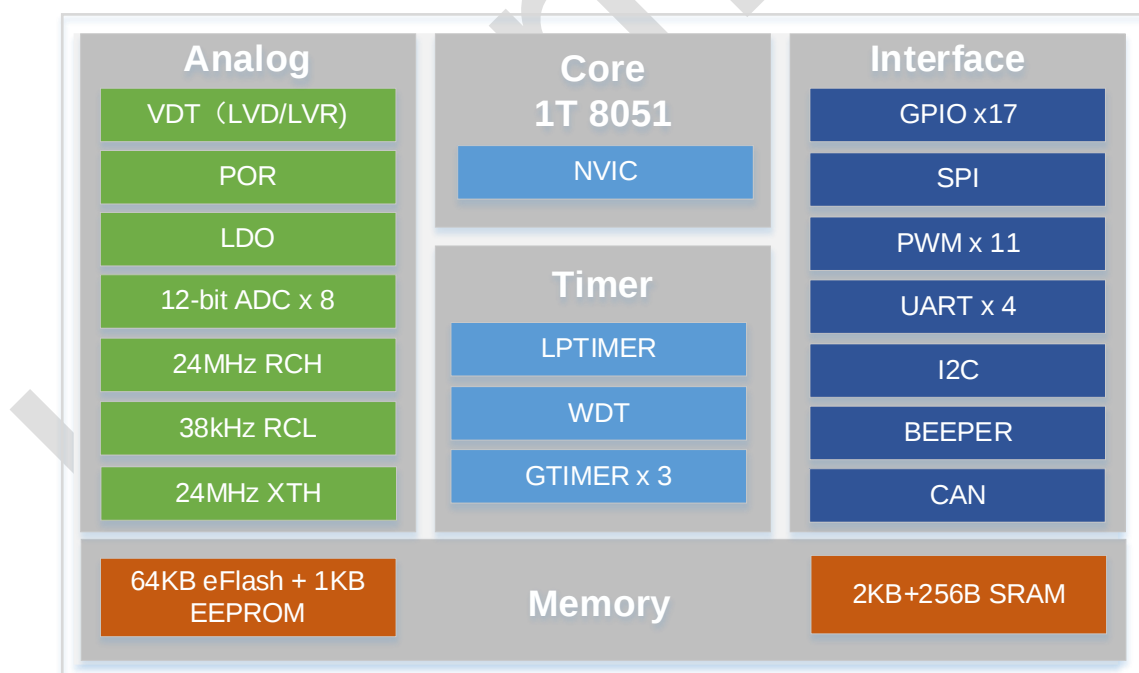
图 1-1：芯片功能图
