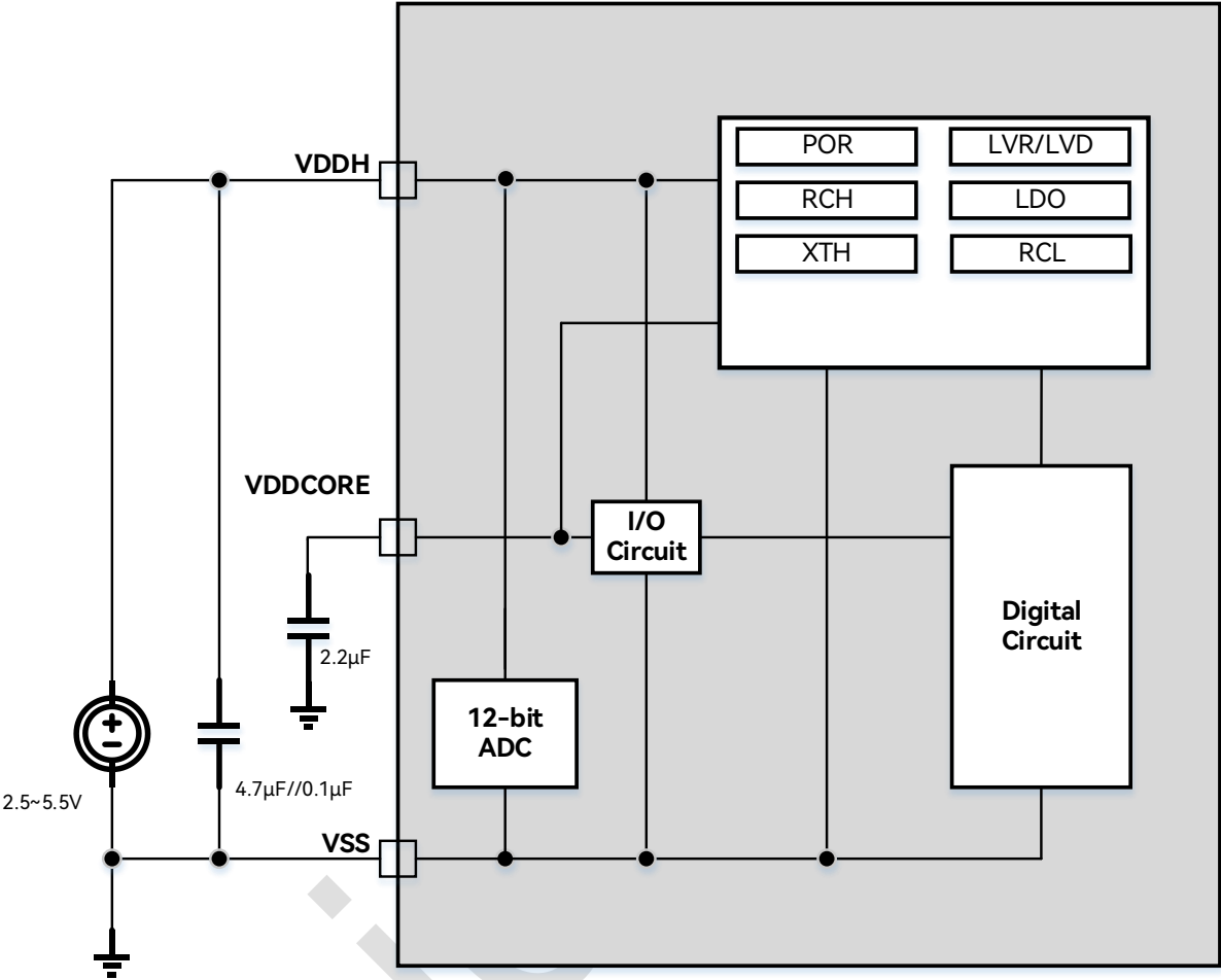
图 20-1：供电方案图
