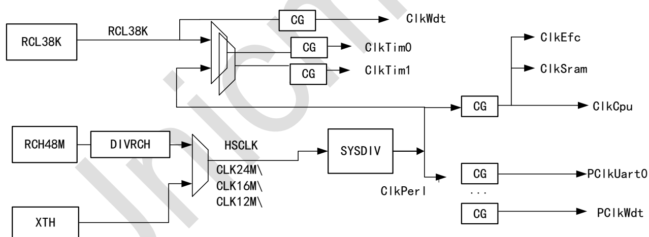
图 4-1：时钟结构图
