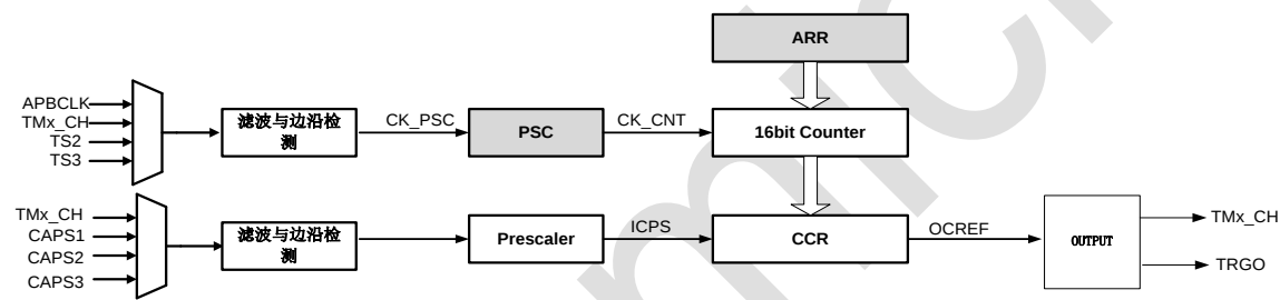
图 13-1：结构框图
