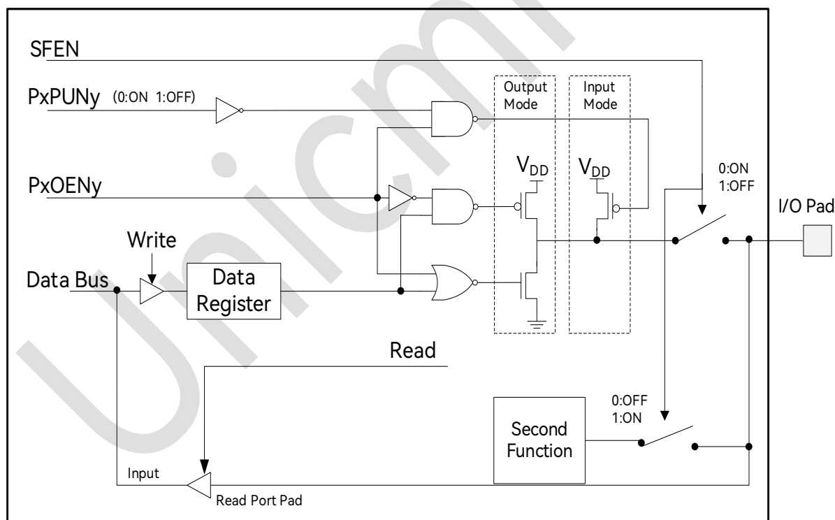
图 7-1: 端口模块图
