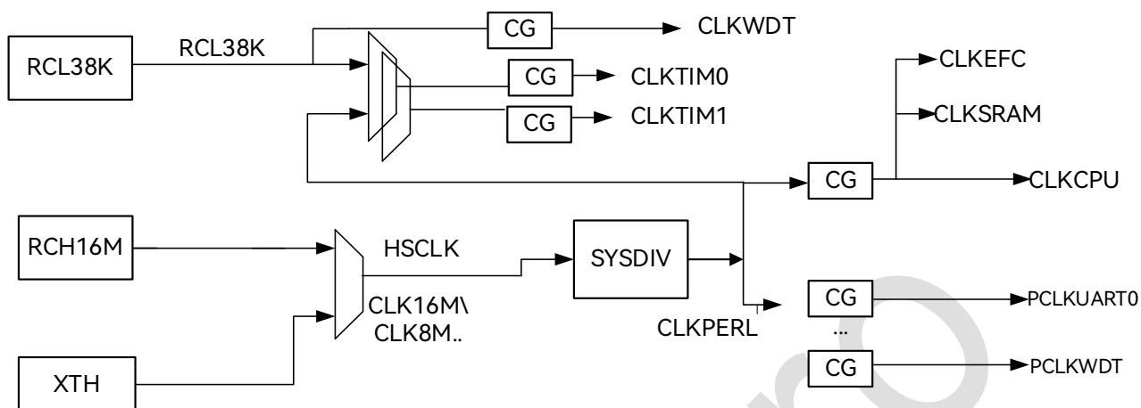
图 4-1: 时钟结构图
