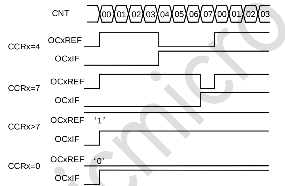
图 13-2: 边沿对齐的 PWM 波形 (ARR=7)
