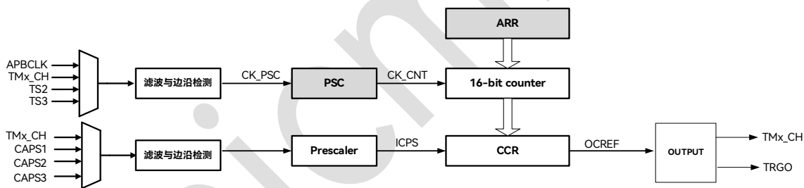
图 13-1：结构框图
