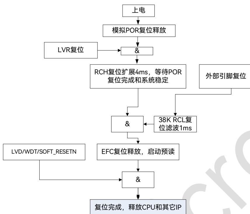
图 4-2: 复位流程图
